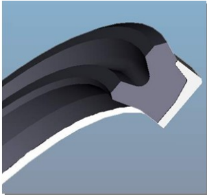
UKL TYPE ROD PACKING
